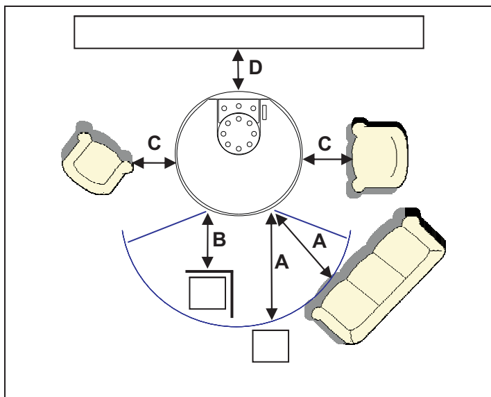
Varnostni odmiki znotraj/izven varnostnega območja pred kuriščem
