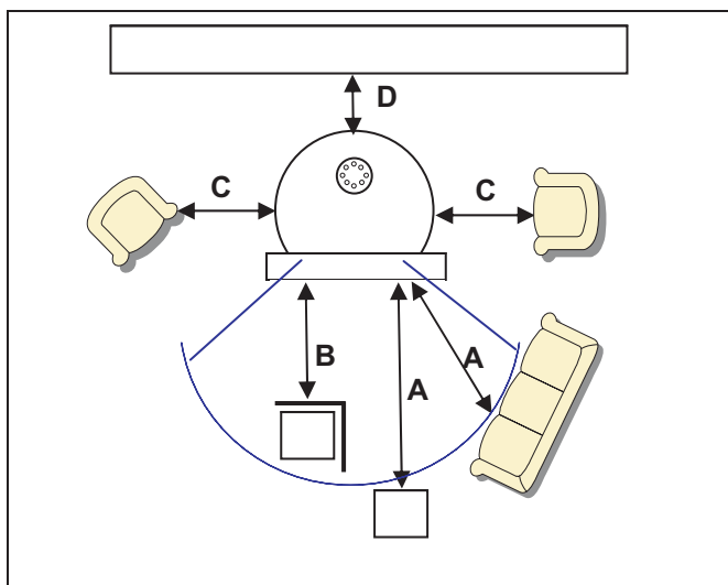
Varnostni odmiki znotraj/izven varnostnega območja pred kuriščem
