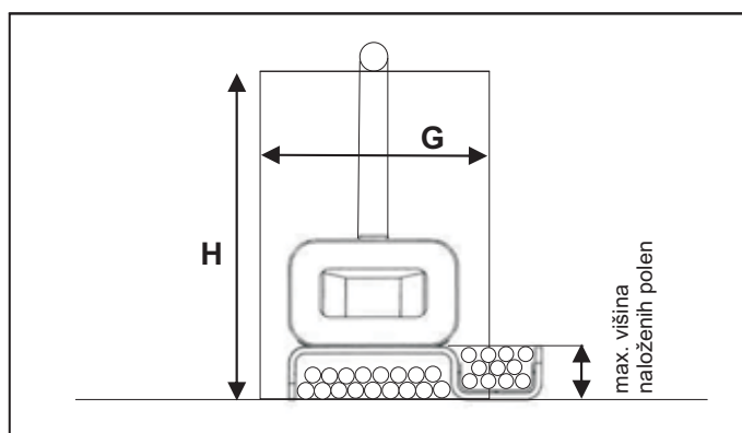
Prezračevana, ognjeodporna zaščita (zaslon) pred sevanjem (npr. iz jeklene pločevine)
