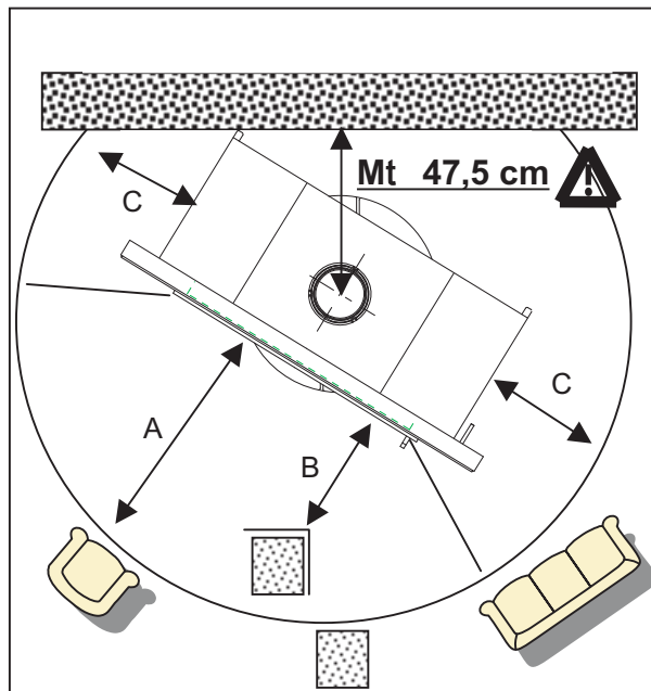
Varnostni odmiki, če se peč vrti
