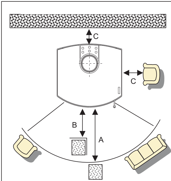
Varnostni odmiki znotraj/izven varnostnega območja pred kuriščem
