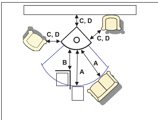
Varnostni odmiki znotraj/izven varnostnega območja pred kuriščem (montaža pred steno)
