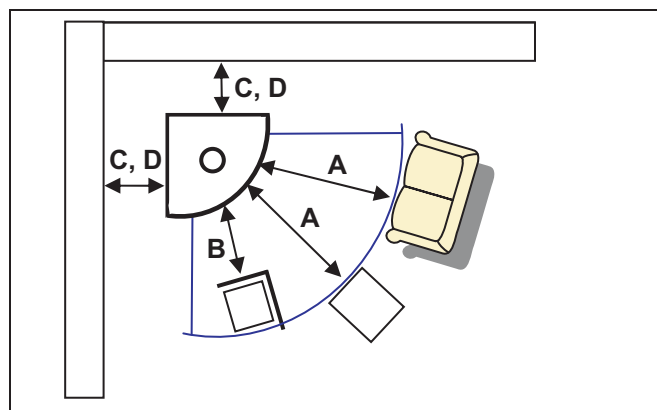
Varnostni odmiki znotraj/izven varnostnega območja pred kuriščem (montaža v kotu)
