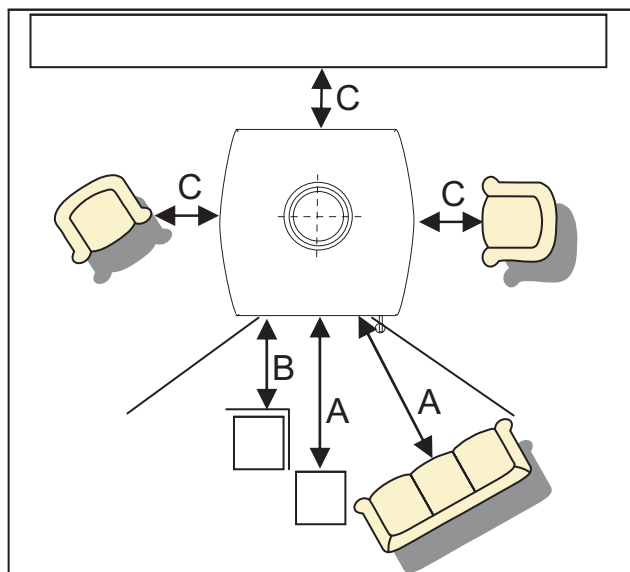
Požarno varnostni odmiki znotraj/izven varnostnega območja pred kuriščem
