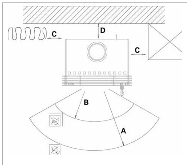
Varnostni odmiki znotraj/izven varnostnega območja pred kuriščem
